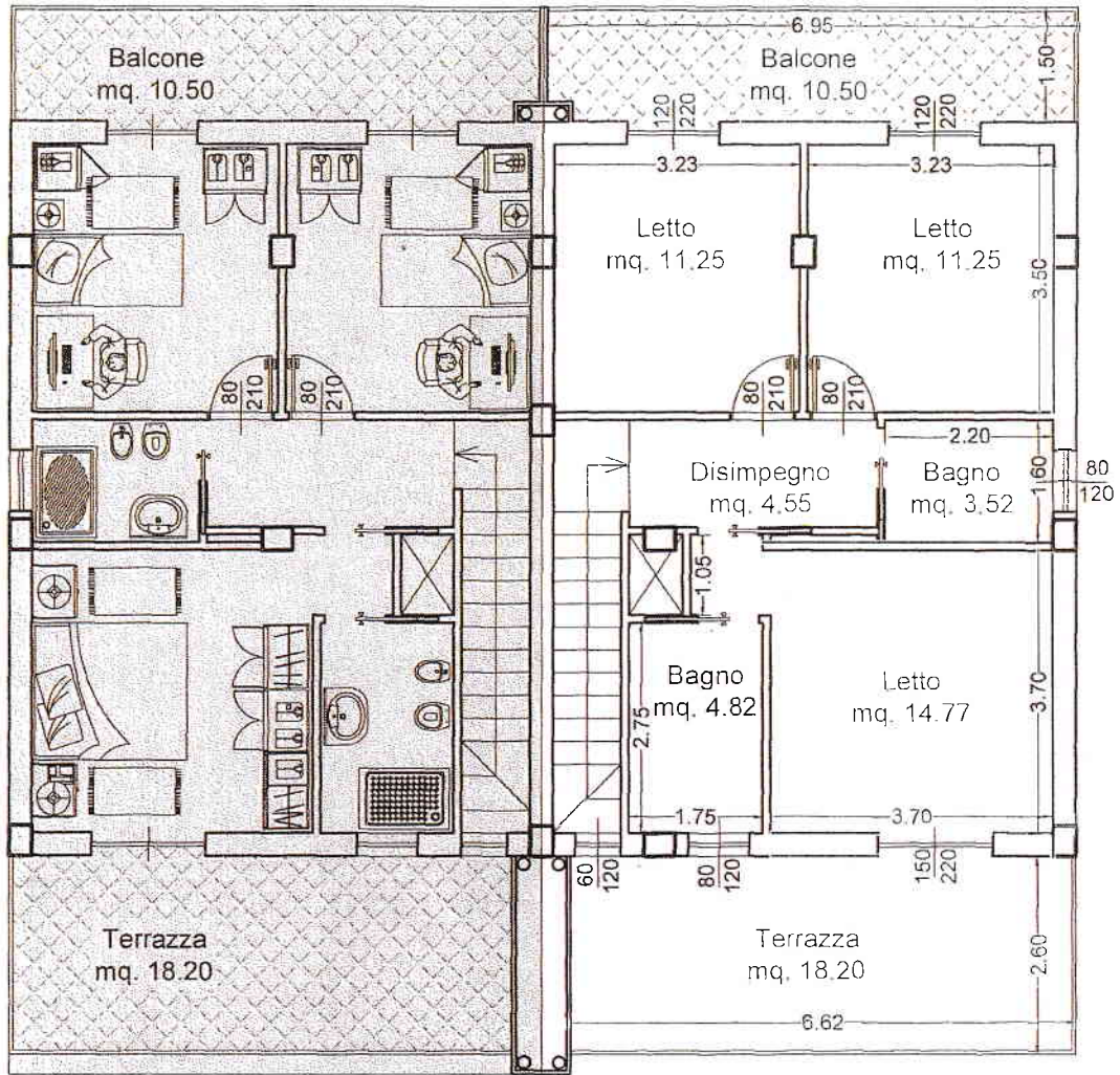
PIANTA PIANO PRIMO -scala 1:100-
